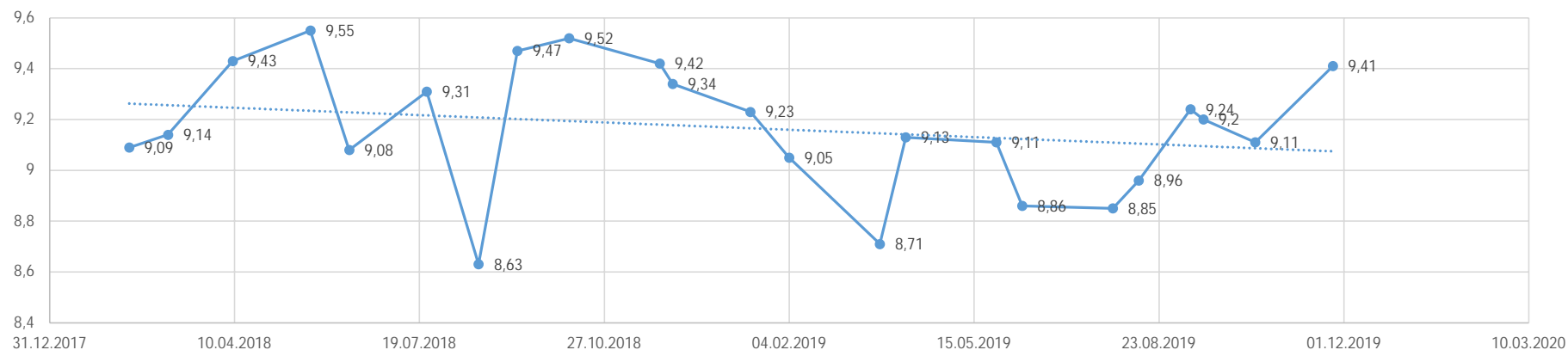
Průběh hodnot pH ve veřejném vodovodu Červený Potok 2017 -2019 se spojnicí trendu
