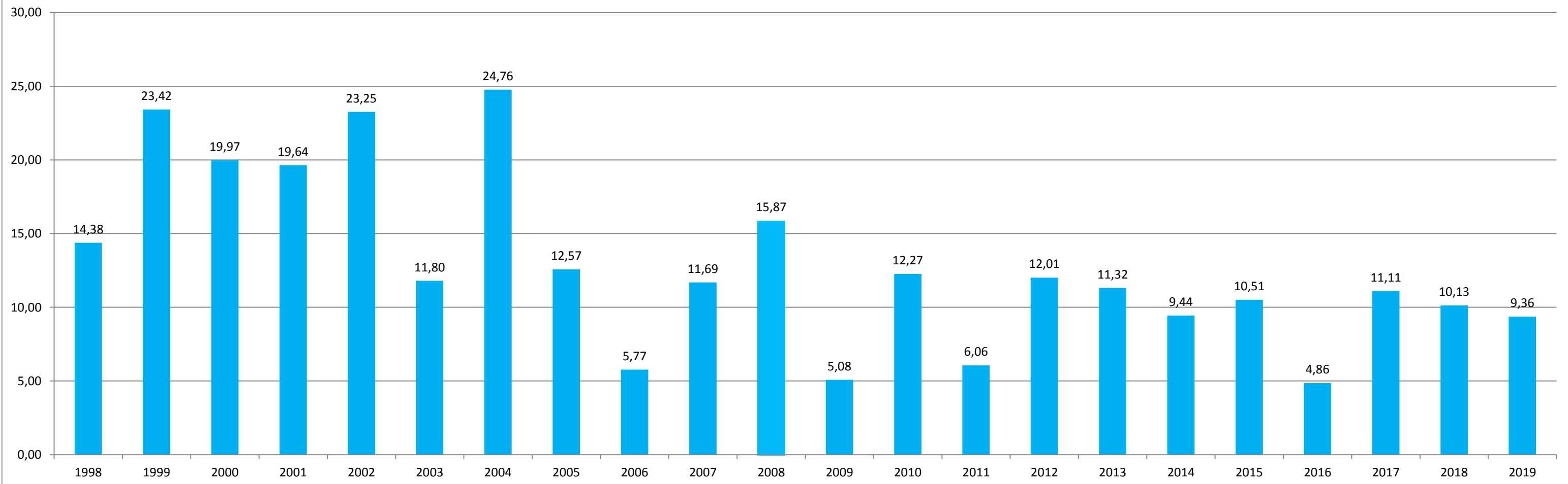
Ztráty ve vodovodní síti v % - provoz vodovodů Choceň
