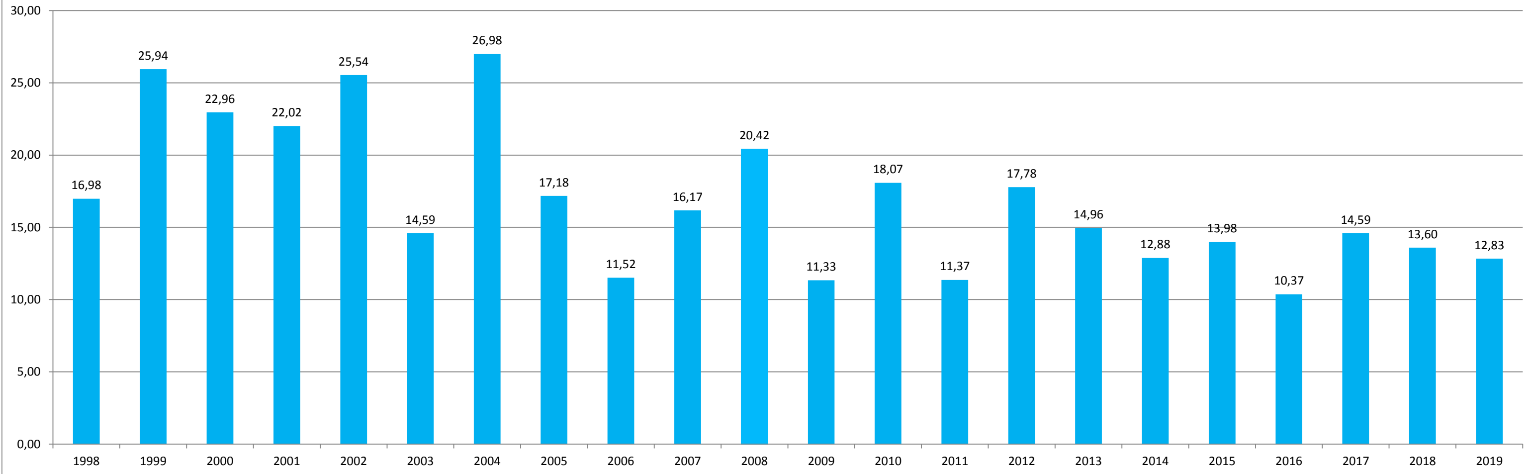
Voda nefakturovaná v % - provoz vodovodů Choceň
