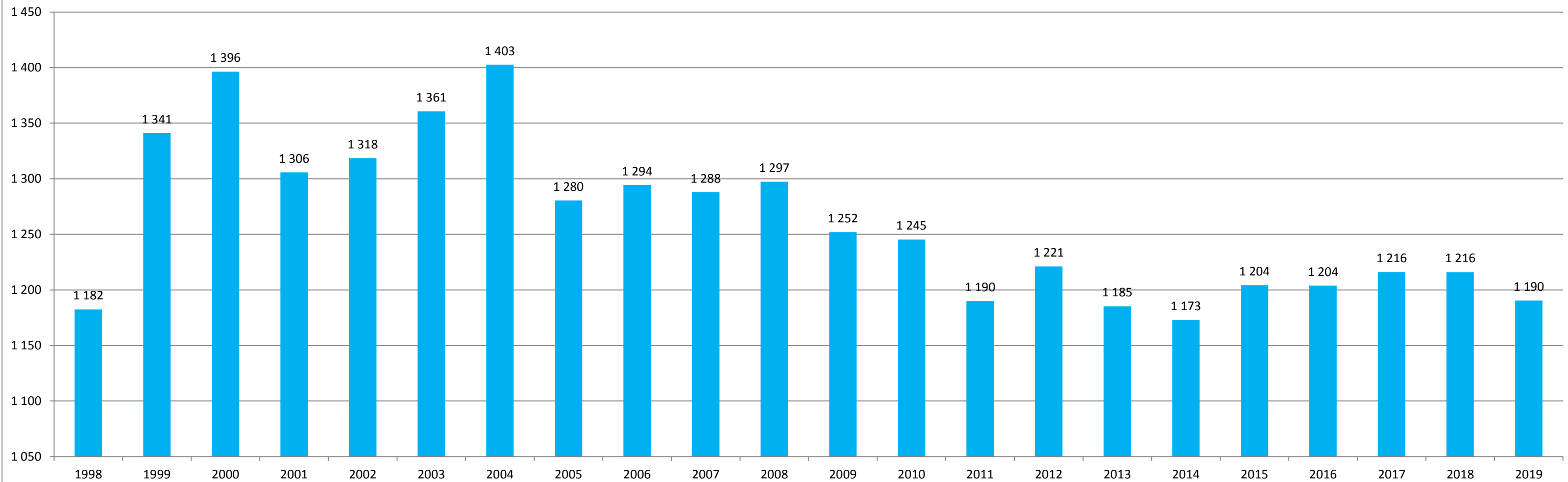
Voda určená k realizaci v tis. m 3 - provoz vodovodů Lanškroun
