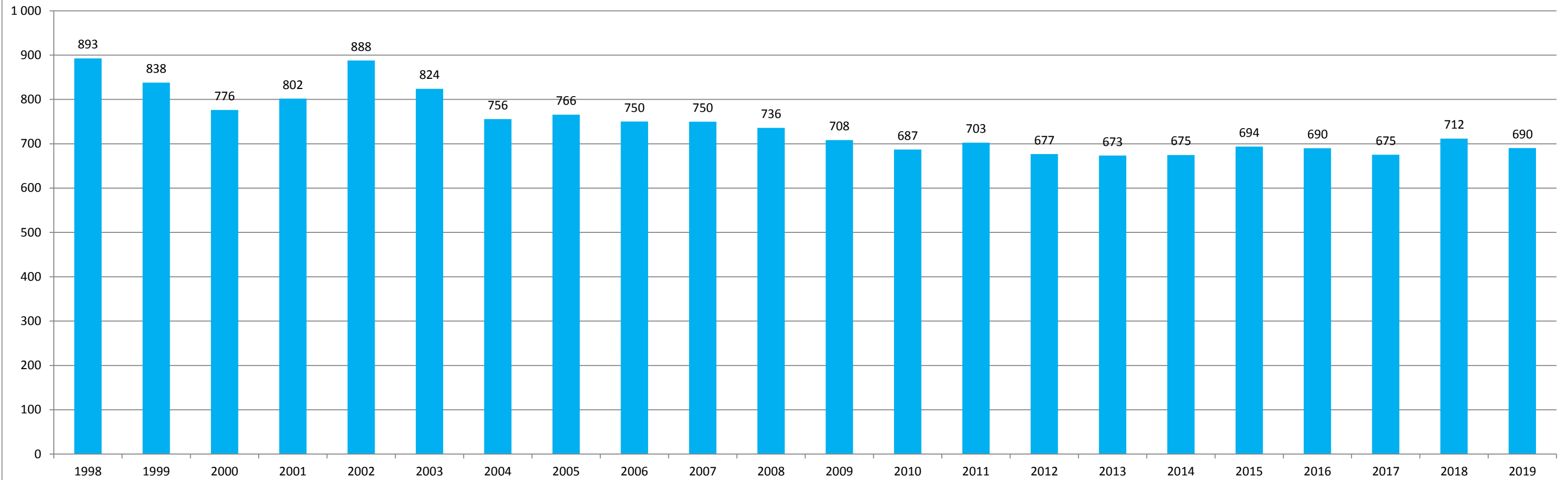
Fakturovaná voda v tis. m 3 - provoz vodovodů Jablonné nad Orlicí
