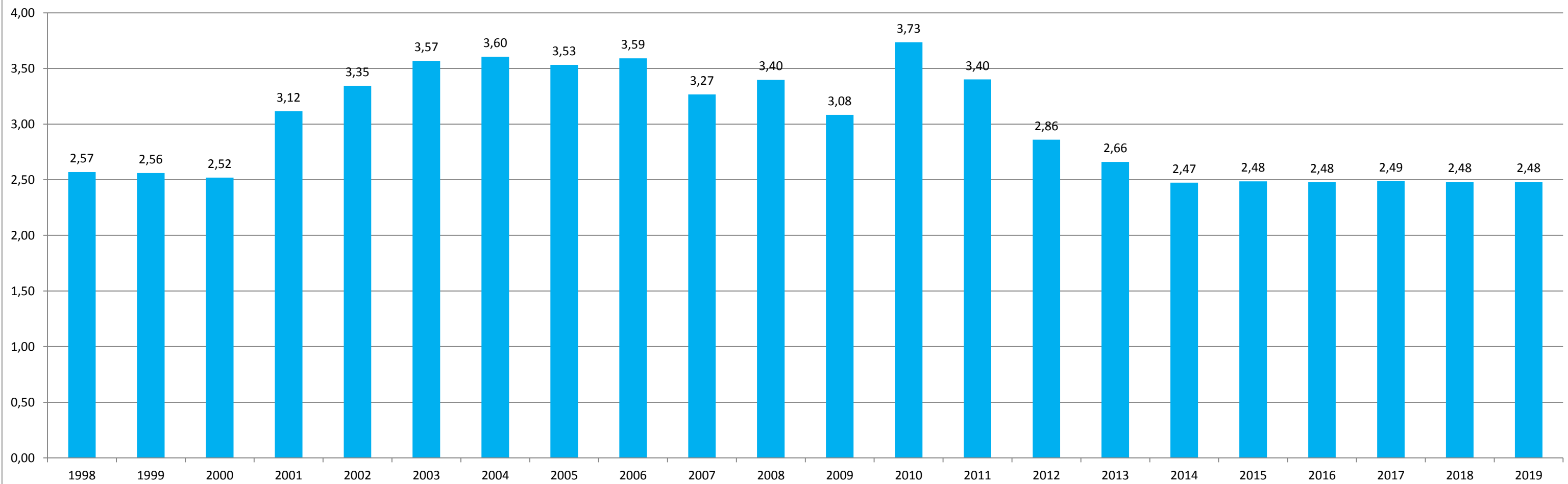
Vlastní spotřeba vody v % - provoz vodovodů Ústí nad Orlicí
