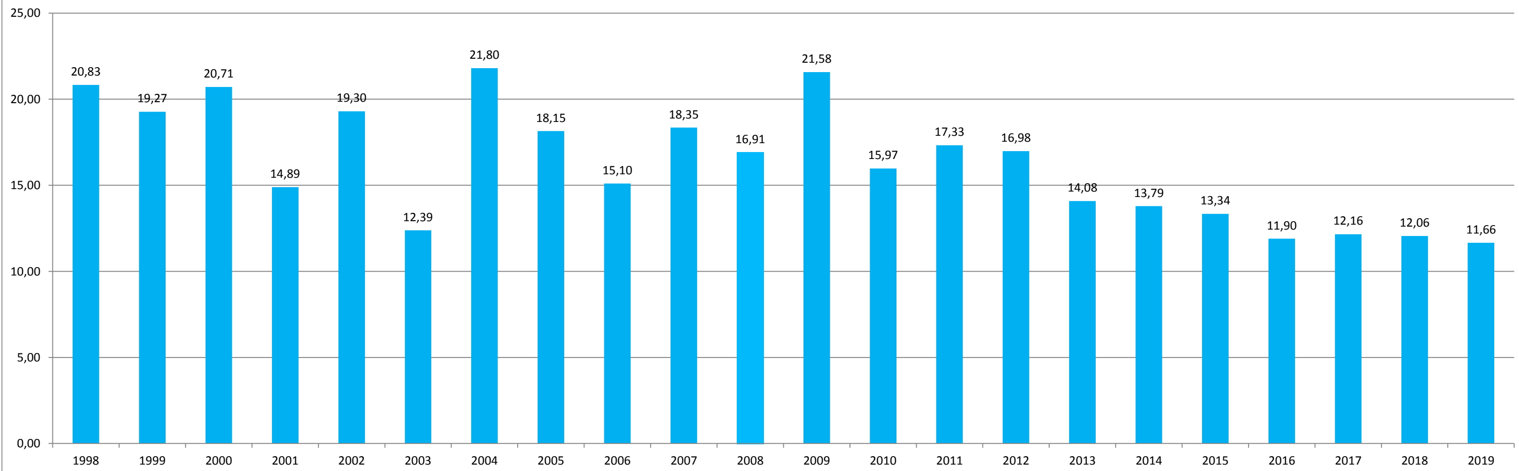
Ztráty ve vodovodní síti v % - provoz vodovodů Ústí nad Orlicí
