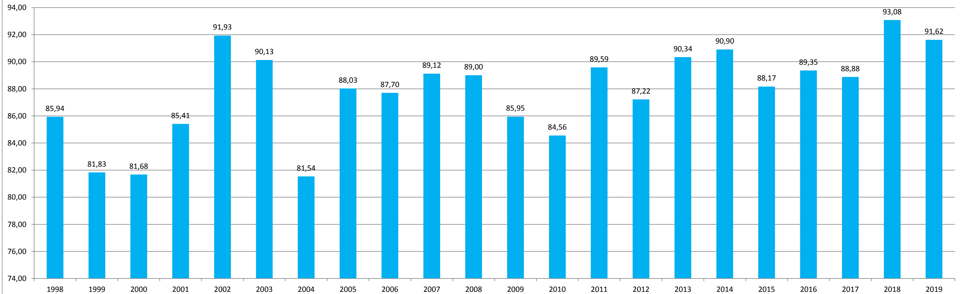
Podíl vody fakturované z vody určené k realizaci v % - provoz vodovodů Lanškroun
